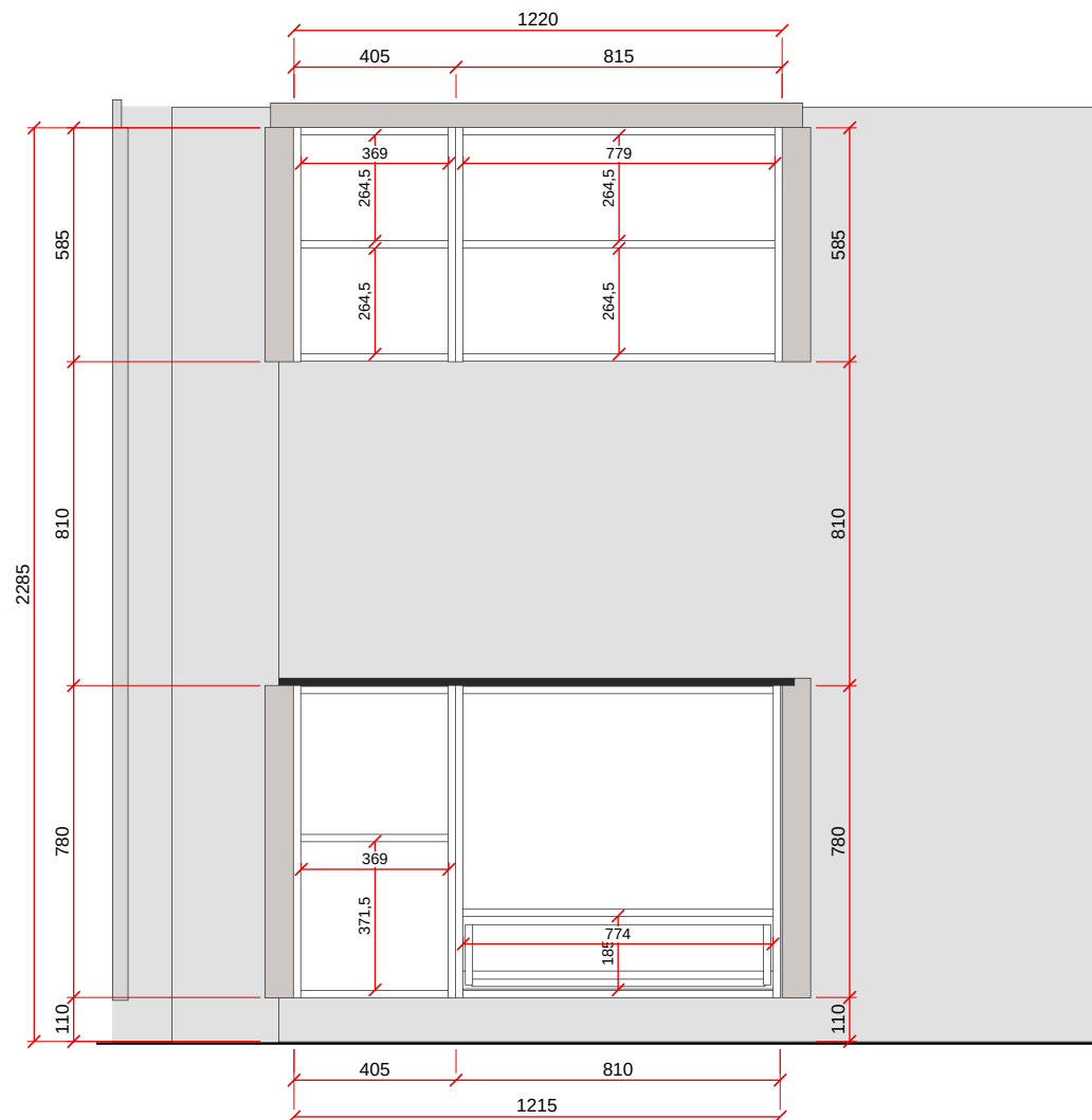
VISTA C - ESC. 1:20
