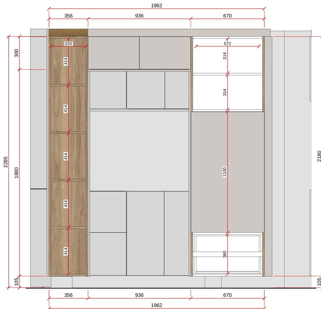
VISTA B - ESC. 1:20
